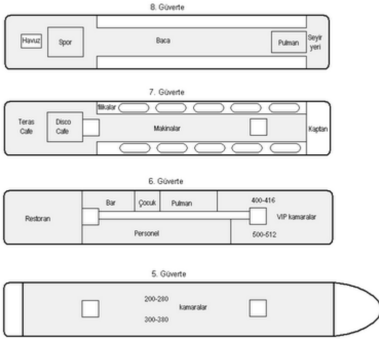
Güverte planı
